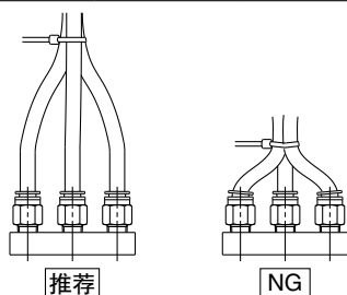
图2 用扎带捆绑配管的场合
