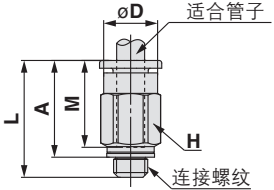
释放套尺寸
