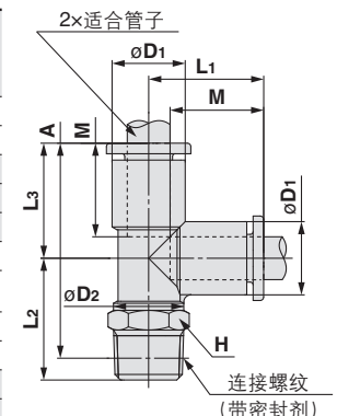
释放套尺寸
