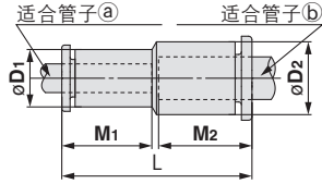
释放套尺寸
