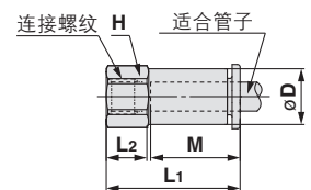
释放套尺寸
