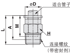
释放套尺寸
