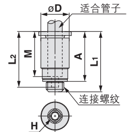
释放套尺寸
