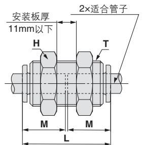
释放套尺寸
