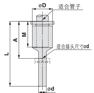
释放套尺寸
