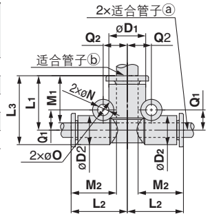
释放套尺寸
