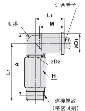
释放套尺寸
