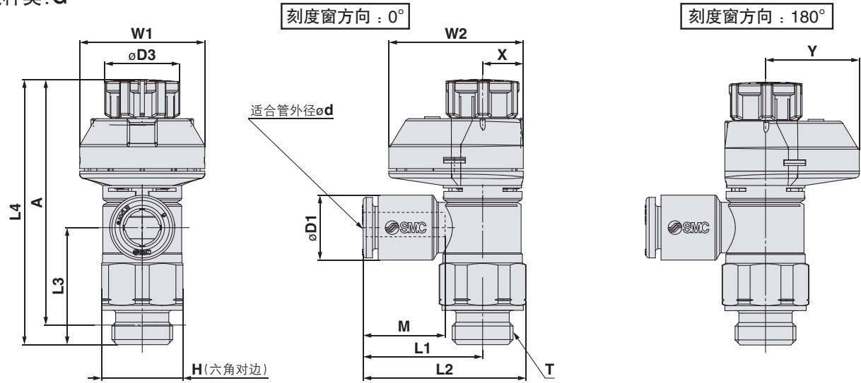
公制尺寸
