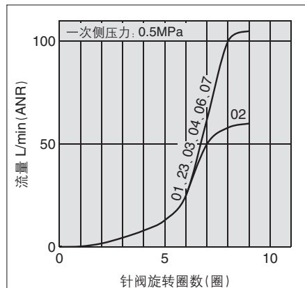
AS1□01FS□-M5□、AS1□11FS□-M5□
