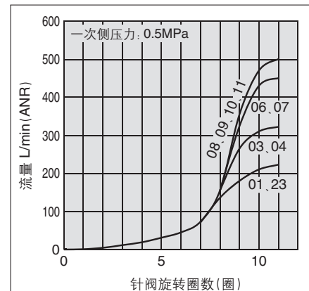
AS2□01FS□-02、AS2□11FS□-02
