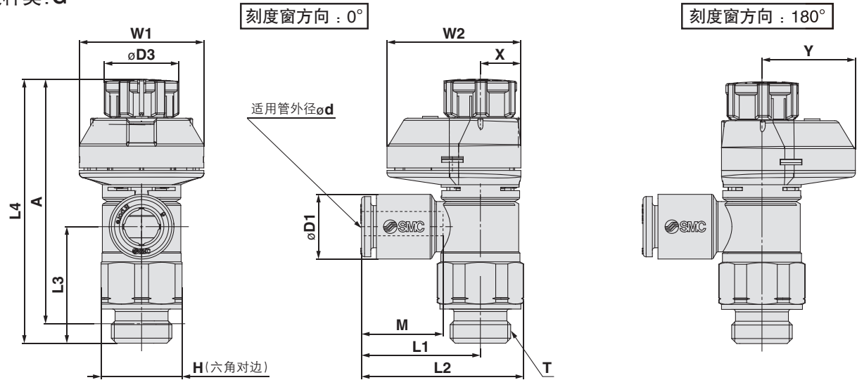
公制尺寸
