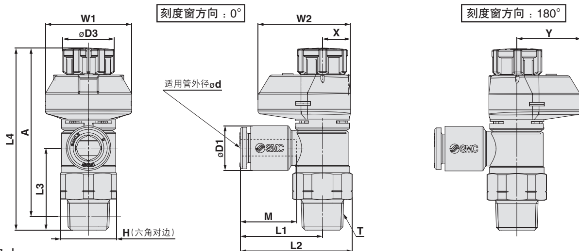
公制尺寸
