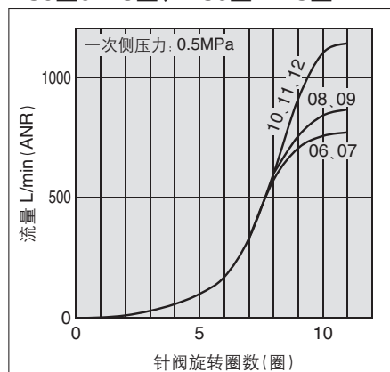
AS3□01FS□、AS3□11FS□
