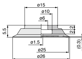
ZP2-B25MT□
