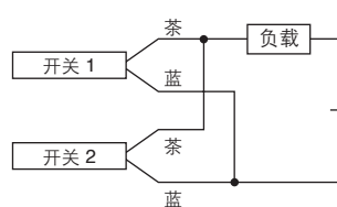
2线式的2个OR连接的场合
