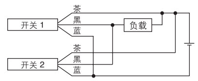
NPN输出的OR连接
