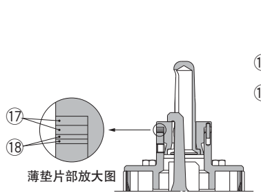
CKQGDA50□-□R□LS 夹紧位置高度: LOW型 带薄垫片的场合
