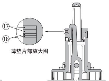
CKQGDA50□-□R□HS 夹紧位置高度: HIGH型 带薄垫片的场合
