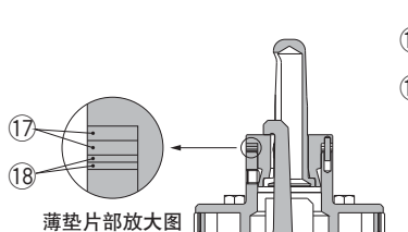
CKQPDA50□-□R□LS 夹紧位置高度: LOW型 带薄垫片的场合
