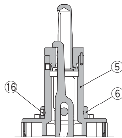
CKQGDA50□-□R□H 夹紧位置高度: HIGH型 无薄垫片的场合
