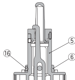
CKQPDA50□-□R□H 夹紧位置高度: HIGH型 无薄垫片的场合
