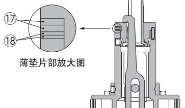
CKQPDA50□-□R□HS 夹紧位置高度: HIGH型 带薄垫片的场合
