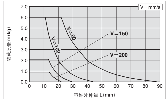
MXQ20(A)-100、150Z□
