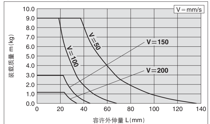
MXQ25(A)-125、150Z□
