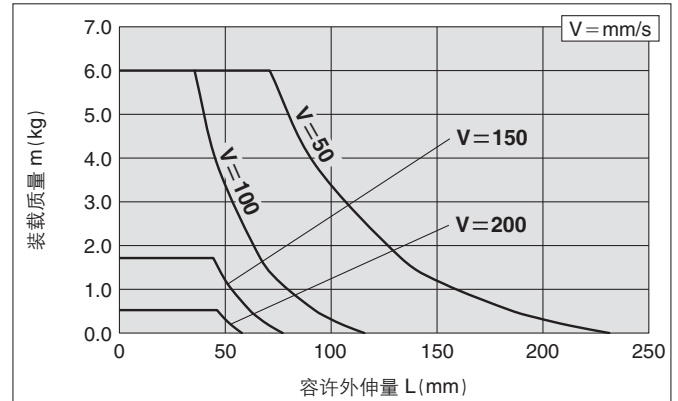
MXQ25(A)-50、75Z□
