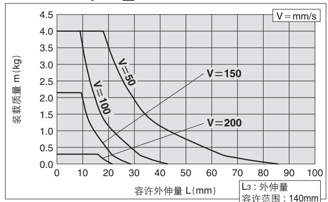
MXQ12B-100、125Z□
