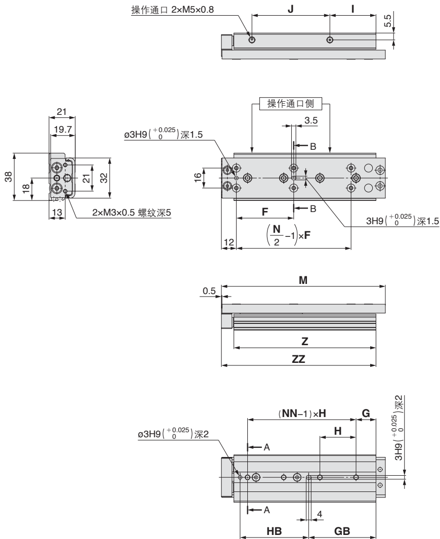
MXQ8C-30Z的底面图
