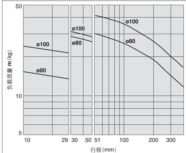
MGPL80 · 100, MGPA80 · 100
