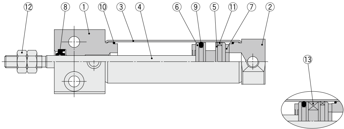
CDJ2RA10, 16-□Z-Bの場合
