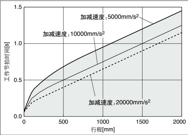
LEJB40 / 同步带驱动
