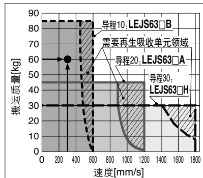
〈速度—搬运质量曲线图〉 (LEJS63)
