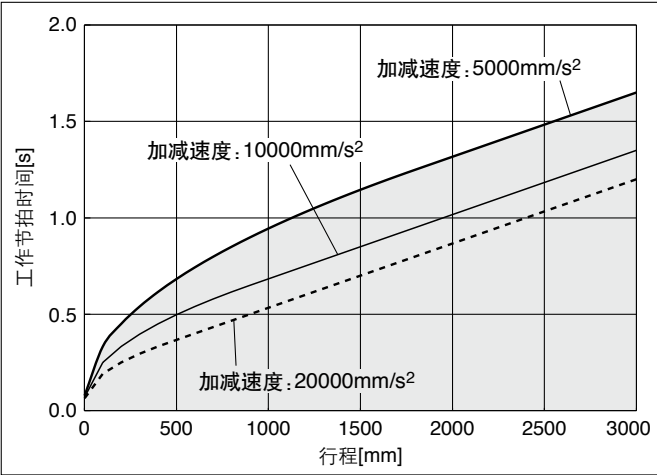
LEJB63 / 同步带驱动
