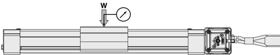
滑台中央有负载重心时
