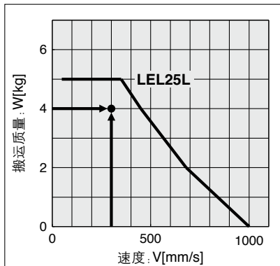
〈速度－可搬质量图〉 (LEL25L / 步进电机)
