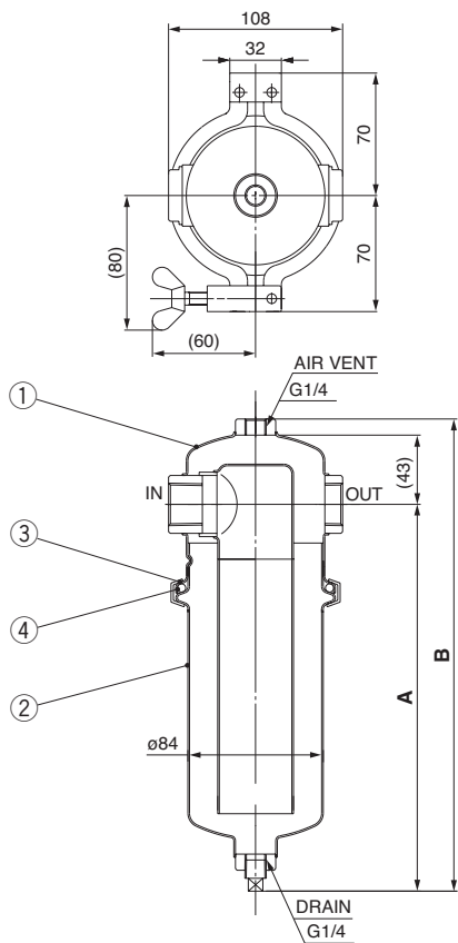
尺寸表 (mm)
