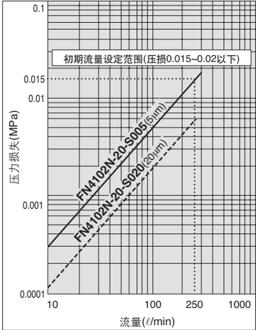
滤芯长度 500ℓ / FN41□2□-20-S□
