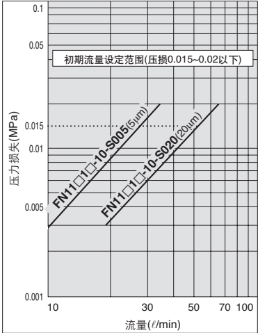
滤芯长度 250ℓ / FN1□□□-10-S□
