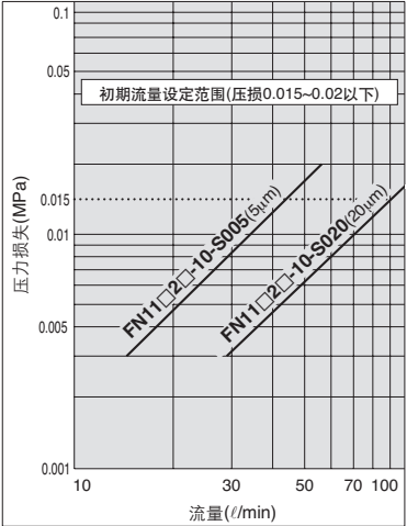
滤芯长度 500ℓ / FN1□2□-10-S□
