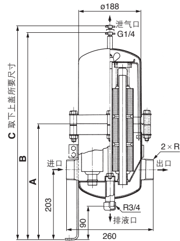
FGET系列(螺钉紧固形式) (mm)
