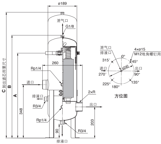
FGES系列(V形带形式) (mm)
